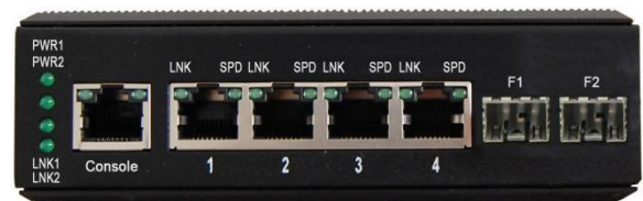
桌面式 千兆 2 光 4 电 交换机
